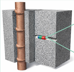
Korrosionsinhibitorn VPI580 Margel™ installeras i 20 mm stora hål som borrar i den betongkonstruktion som ska skyddas
